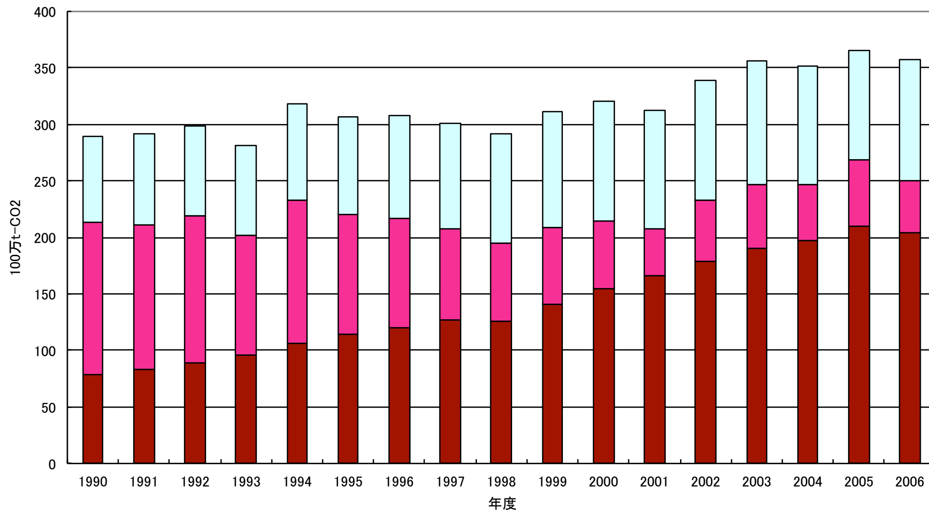
火力発電所(事業用)からの二酸化炭素排出量(1990~2006)
